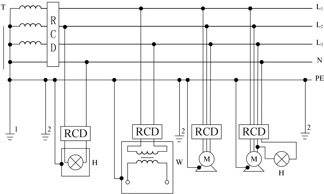
图 3.3.6-1 专用变压器供电 TN-S 系统
